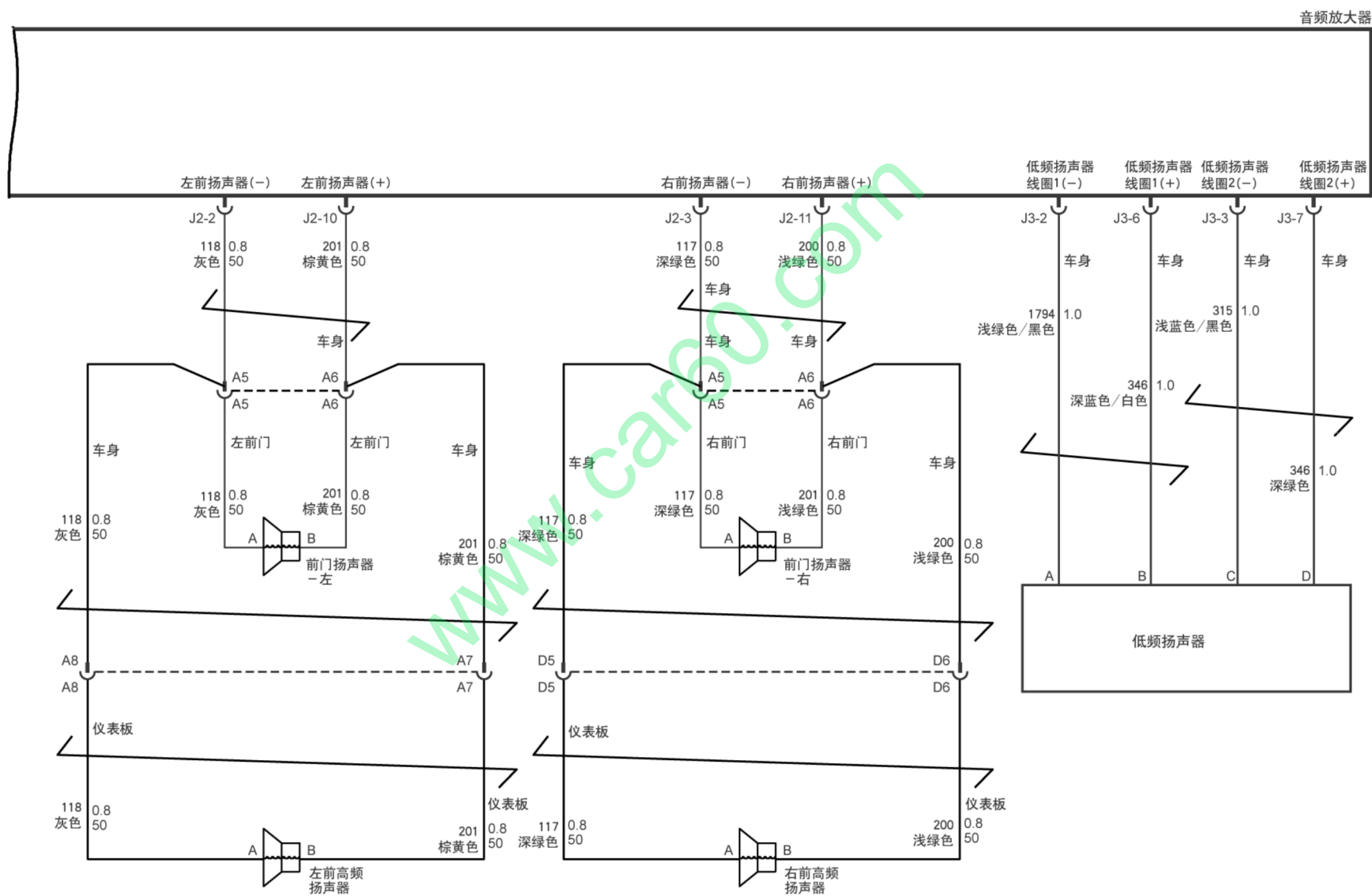
NAVI及娱乐系统扬声器示意图(2-2)
